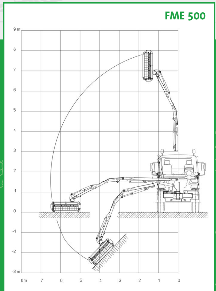
Reichweitendiagramm des FME 500
