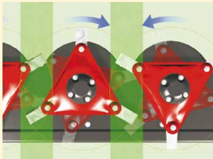
Breite Überlappung dank gegenläufiger Mähscheiben sowie einer geraden Anzahl an dreieckigen Mähscheiben.
