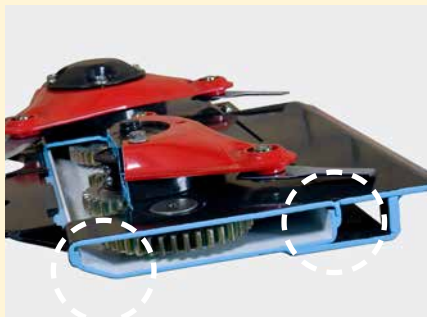
Rundum verschweißter Mähbalken mit überlappenden C-Profilen für äußerst hohe Stabilität und Steifigkeit.
