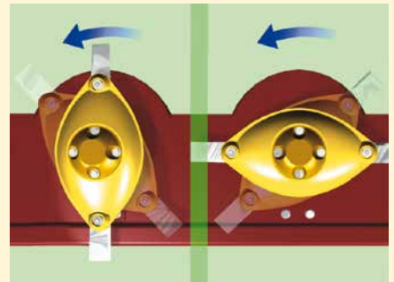
Geringere Überlappung aufgrund ungerader Anzahl von Mähscheiben welche sich in eine Richtung drehen.
